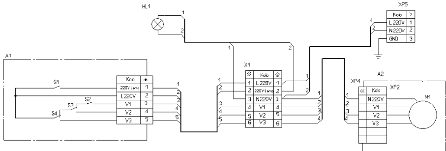
Електросхема принципова витяжки GS Электросхема принципиальная вытяжки GS
