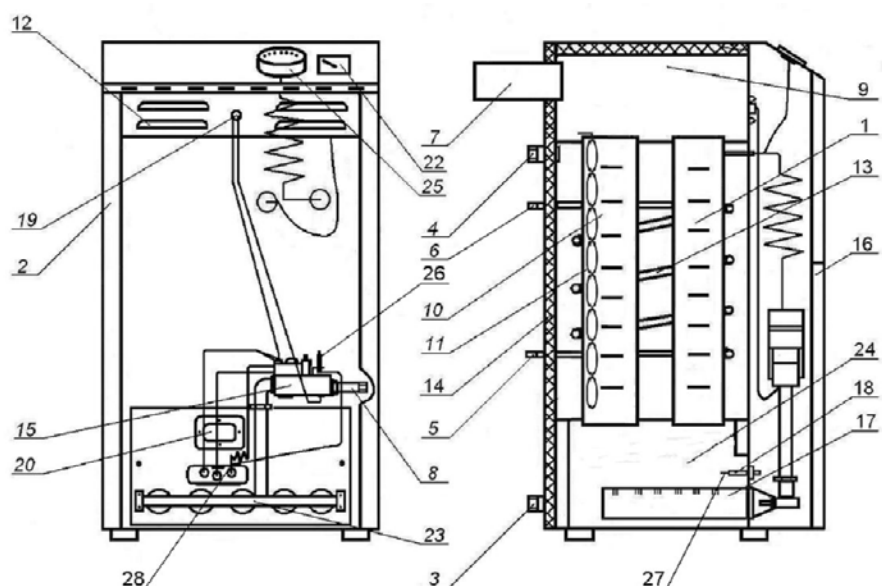
Малюнок 2 - Схема апарата АОГВД-30 ЕВ.
